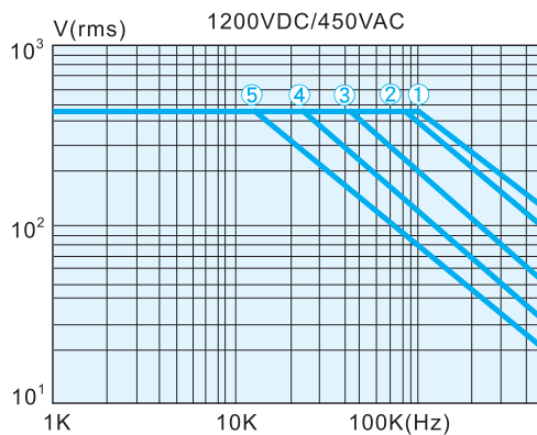
Curve:①.0056 μF ②.01 μF ③.022 μF ④.047 μF ⑤.12 μF
