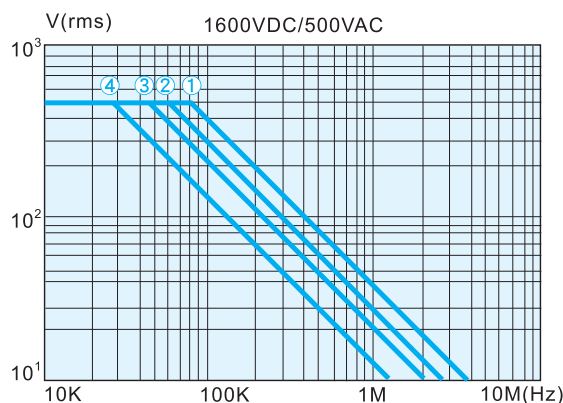
Curve:①.001 μF ②.0056 μF ③.01 μF ④.047 μF
