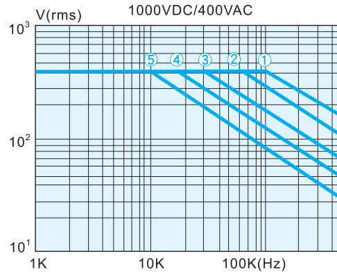
Curve:①.0056 μF ②.01 μF ③.022 μF ④.047 μF ⑤.1 μF
