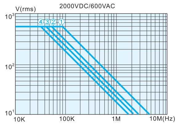
Curve:①.001 μF ②.0047 μF ③.01 μF ④.015 μF
